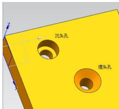
加工図
